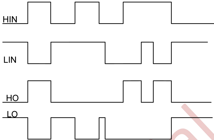
图 9-1 G2021Q 输入输出时序波形
