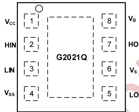
图 7-1 8-脚 DFN 顶视图
